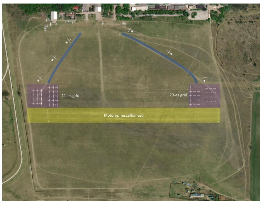
4. ábra. Gridre vontatás útvonala (kék színnel jelölve) 11-es és 29-es pálya szerint. A 11/29-es rajtrácsok helye zölddel, a vontatógép leszállómező sárga színnel jelölve.
