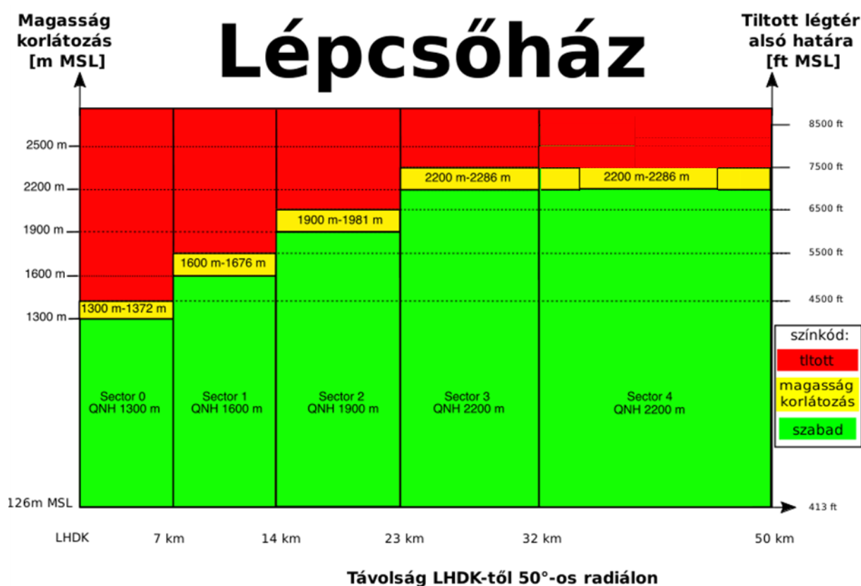
13. ábra. Magasságkorlátozások vertikális metszete.
