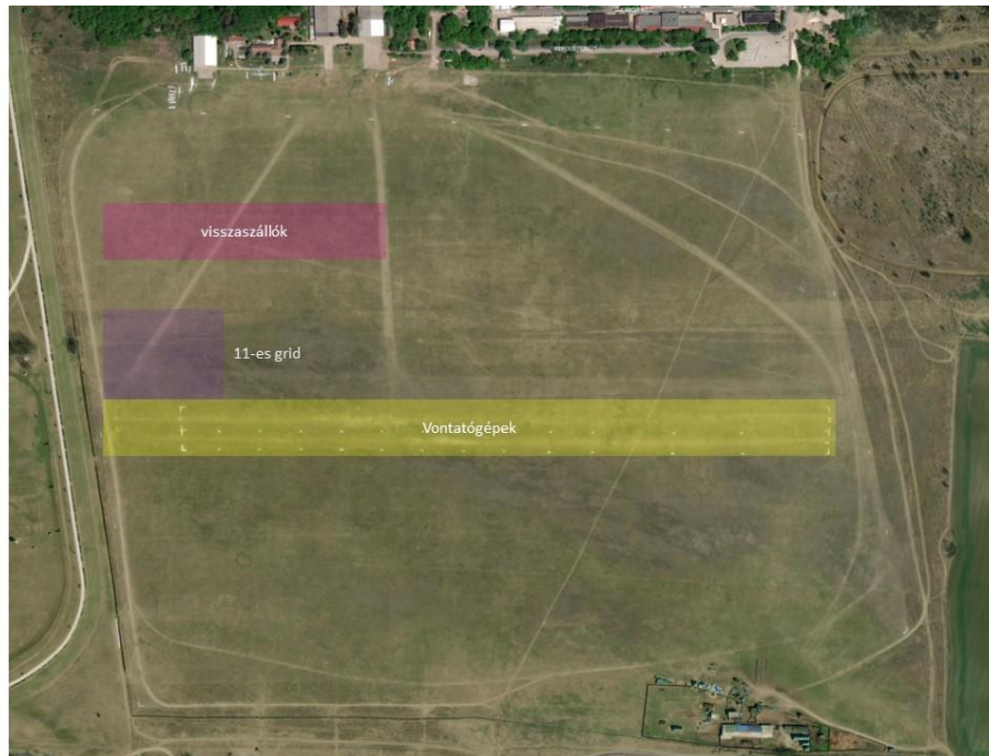
5. ábra. Startberendezés 11-es pálya esetén. A rajtrács zöld, a vontatógép leszállómező sárga, a vitorlázó repülőgép leszállómező (a felvontatás alatt visszaszálló gépeknek) lila színnel jelölve.
