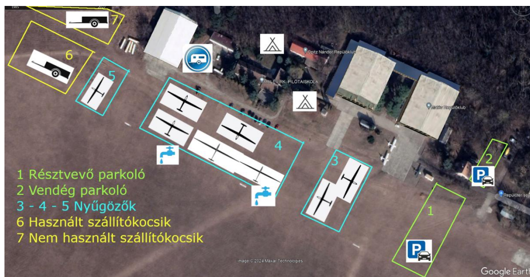
2. ábra: A verseny helyszíne, a parkolók, nyűgözők és a víztöltő állomások elhelyezkedése a repülőtéren
