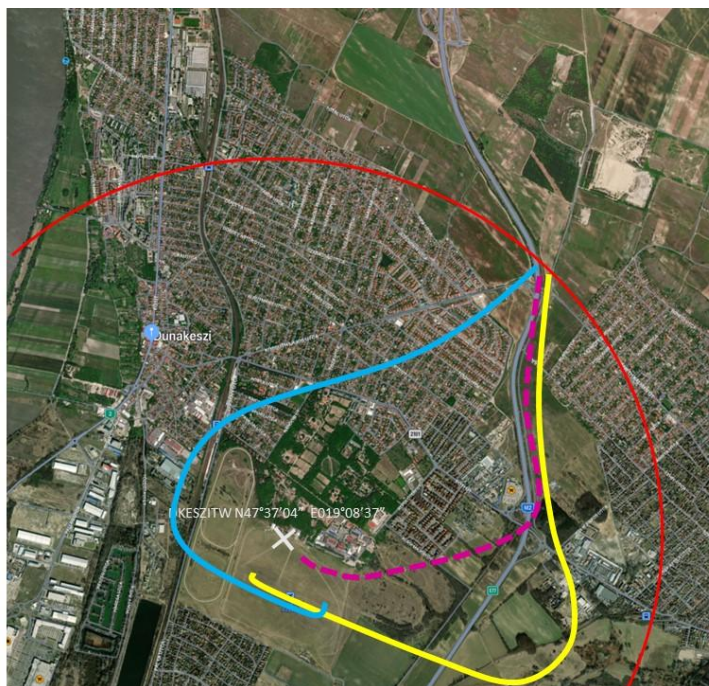
9. ábra: Érkezési eljárások. RWY29 szerint (sárga útvonal), RWY11 szerint (ciánnék útvonal). Érkezés kis energiával (szaggatott magenta színnel jelölt vonalon).
